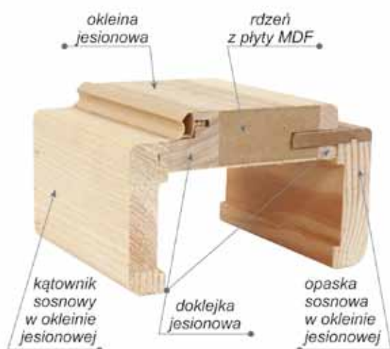
OŚCIEŻNICA W OKLEINIE JESIONOWEJ
